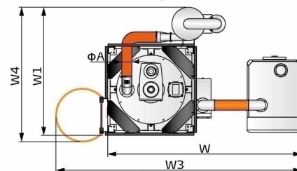
SCR-900U (лестница для тех.обслуживания является опцией)
