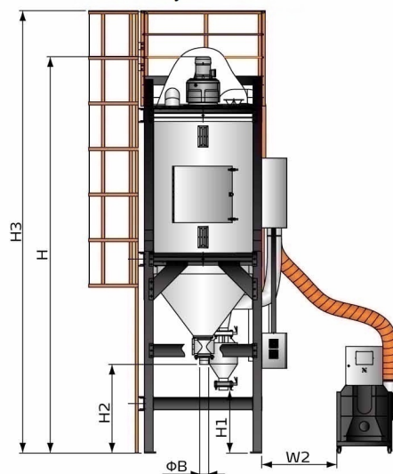
SCR-900U (лестница для тех.обслуживания является опцией)
