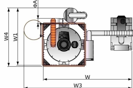
SCR-2500U (лестница для тех.обслуживания является опцией)
